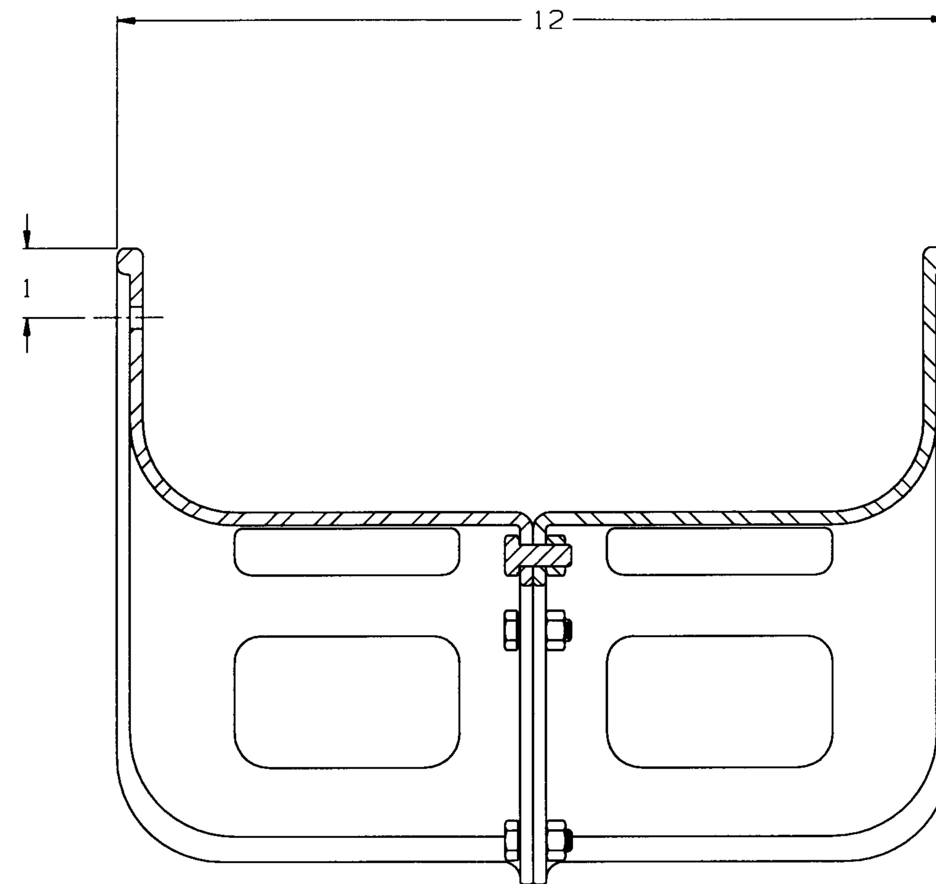
SECTION A-A
